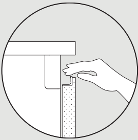
apertura con gola piatta / profilo L90 opening with flat groove and L90 profile
