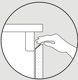
apertura con gola piatta / profilo L40 opening with flat groove and L40 profile
